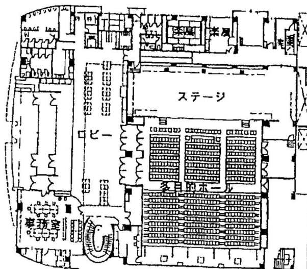
1階平面図
