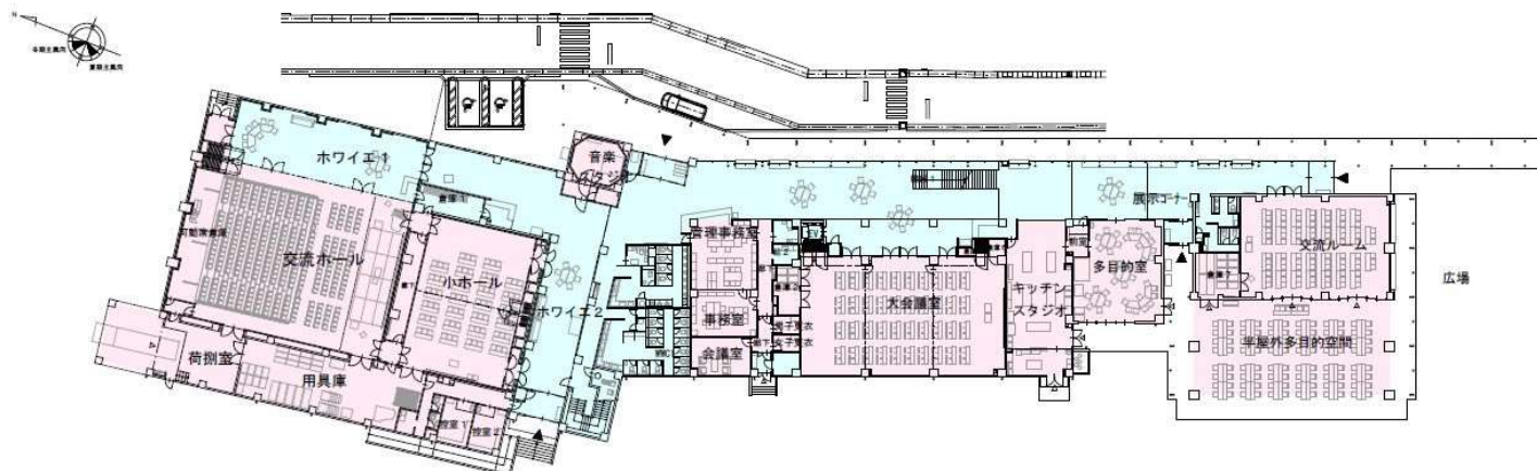
〔1階平面図〕 1:400
