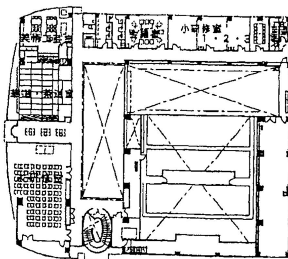
3階平面図
