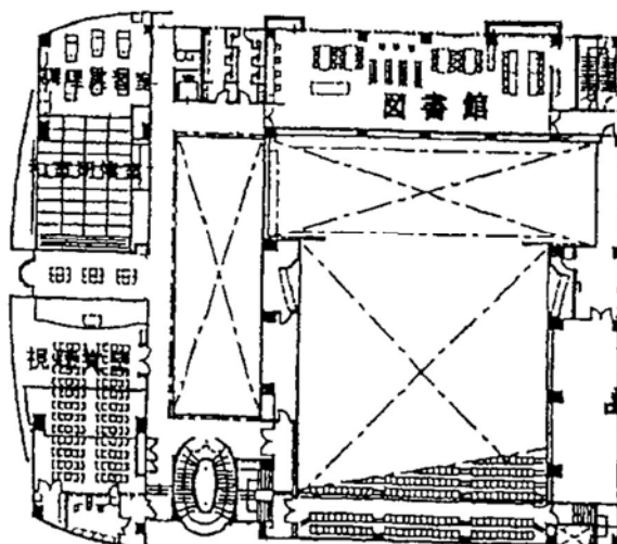
2階平面図
